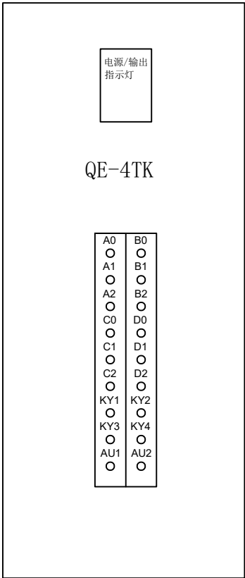
接线示意图
