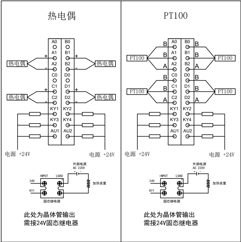
接线示意图
