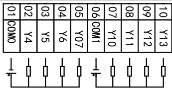
4.3寸一体机MM_20MT_6MT_430A_FX_A接线图
